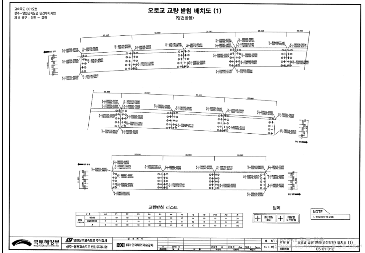
【그림 9.1.5】 교량받침 배치도
