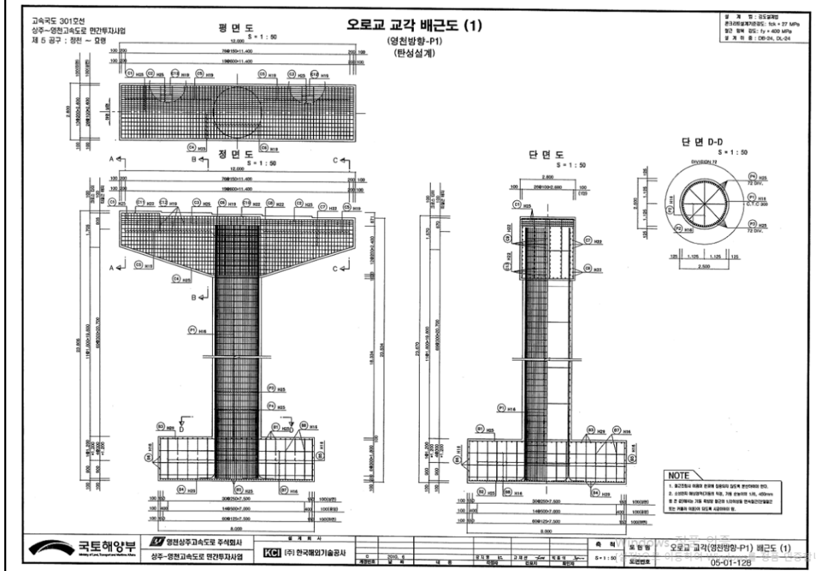
【그림 9.1.10】 교각 배근도
