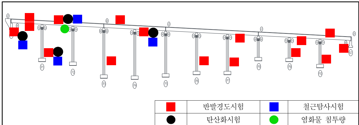
【그림 9.4.1】 콘크리트 내구성조사 위치도(상주방향)
