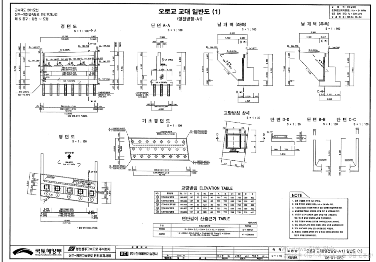
【그림 9.1.6】 교대 일반도
